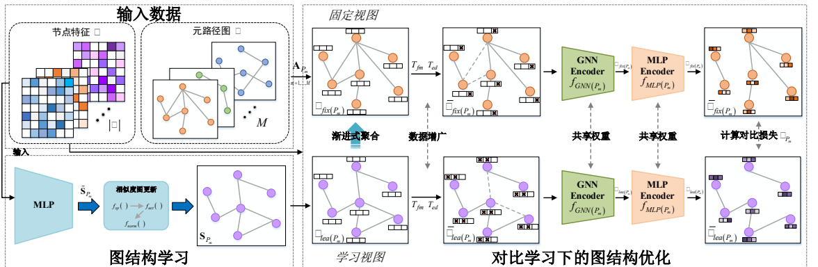
图 4 MV-HGSL 模型框架图
