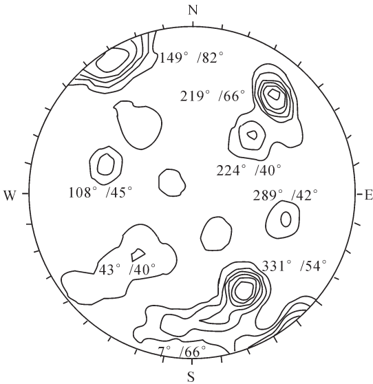
图 4 节理赤平投影求解优势产状图
