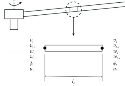
图3 桨叶有限单元节点自由度 Fig. 3 Blade finite element node freedom
