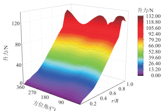
图6 气动载荷随展向一周向分布图
