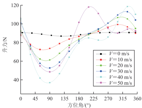
图5 气动载荷随方位角分布图
