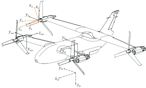
图1 倾转四旋翼机 [15]
