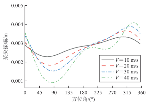
图9 前飞过程桨叶振动响应
