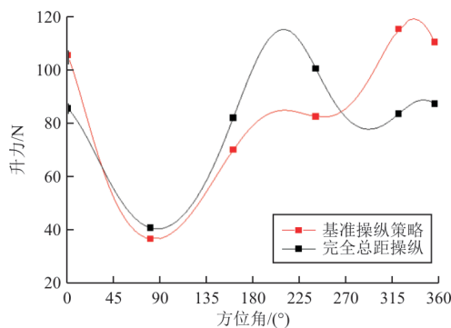
图7 不同操纵策略下气动载荷随方位角分布图
