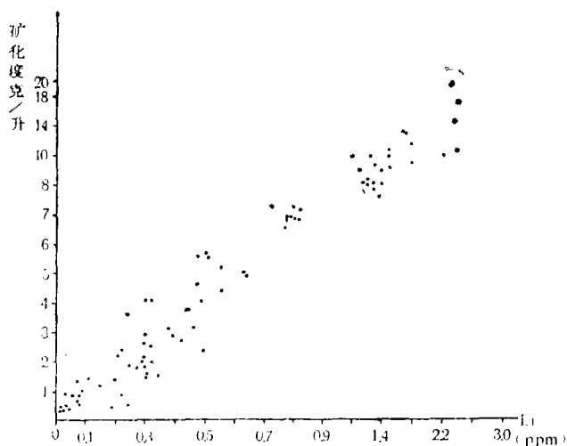
图 4 Li-矿化度的相关性表
