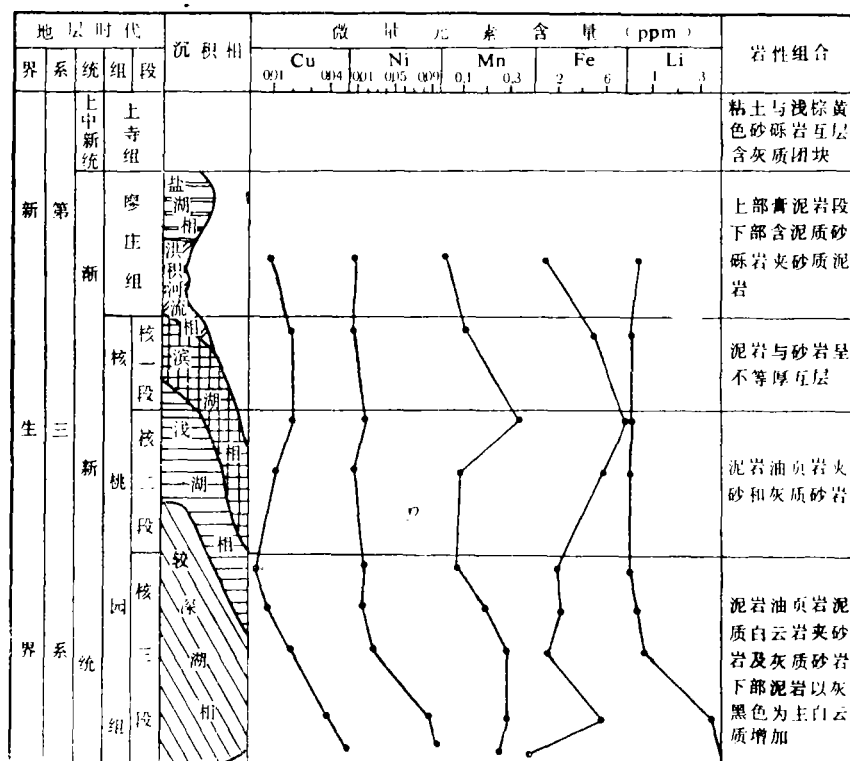
图1 泌阳凹陷沉积特征与微量元素分布图
