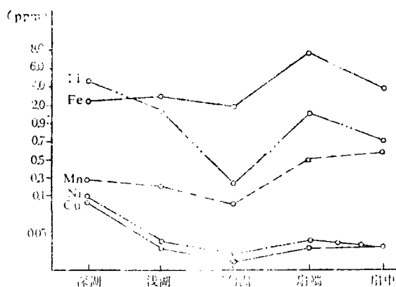
图2 微量元素在各沉积相的含量变化图
