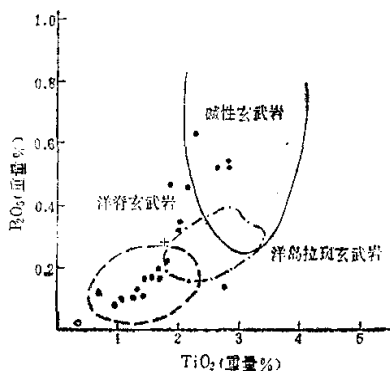
图5 巴音沟蛇绿岩基性熔岩 TiO_2 - P_2O_5 相关图(据 Bass et al., 1973, 转引自王希斌等, 1984, 图1) Fig. 6 TiO_2 - P_2O_5 diagram of basaltic lavas from Bayingol ophiolitic suite
