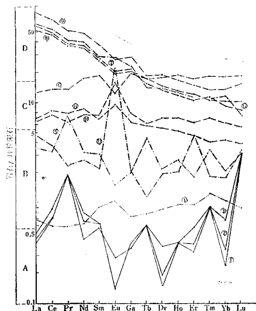
图6 巴音沟蛇绿岩套各类岩石的稀土元素分配模式 (标准化值采用Langmuir et al., 1984)
