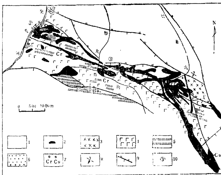
图2 巴音沟—奎屯河一带蛇绿岩分布简图
