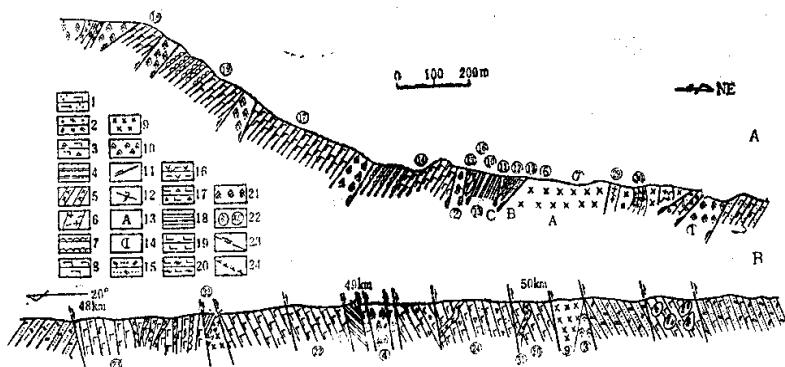
图3 巴音沟(A)和独库公路奎屯河段(B)蛇绿岩实测剖面图
