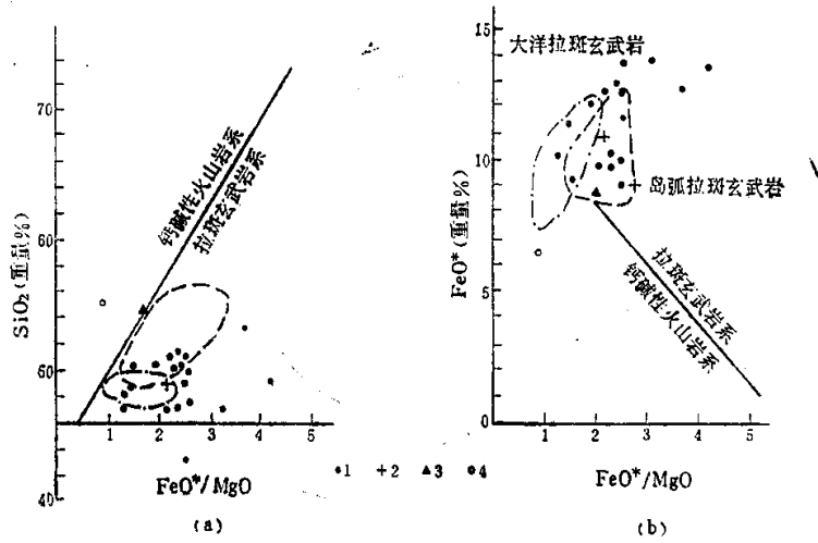
图 4 巴音沟蛇绿岩基性熔岩 \text{FeO}^*/\text{MgO} 值对 \text{SiO}_2 (a)和 \text{FeO}^* (b)的变异图(引自从柏林(1979, p237)) 1. 本区基性熔岩; 2. 本区基性熔岩平均值; 3. 西藏日喀则蛇绿岩基性熔岩平均值(郑万明等, 1984); 4. 阿曼塞迈尔蛇绿岩基性熔岩平均值(科尔曼, 1977, 表7.9) Fig. 5 \text{SiO}_2 - \text{FeO}^*/\text{MgO} and \text{FeO}^* - \text{FeO}^*/\text{MgO} diagrams of basaltic lavas from Bayingol ophiolitic suite
