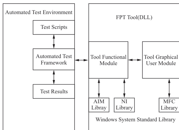
图2 工具架构
