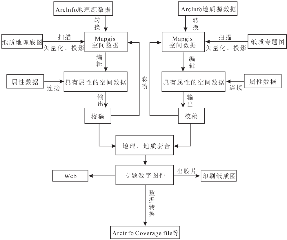
图 1 地质图编制流程图
