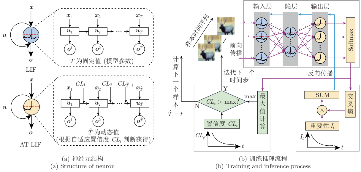
图1 ATSNN 结构及训练和动态时间推理流程图
