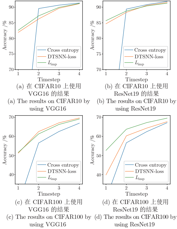
图 4 固定时间步时使用三种损失函数的准确率
