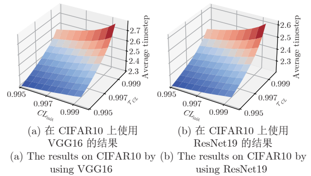
图 6 超参数对时间步的影响
