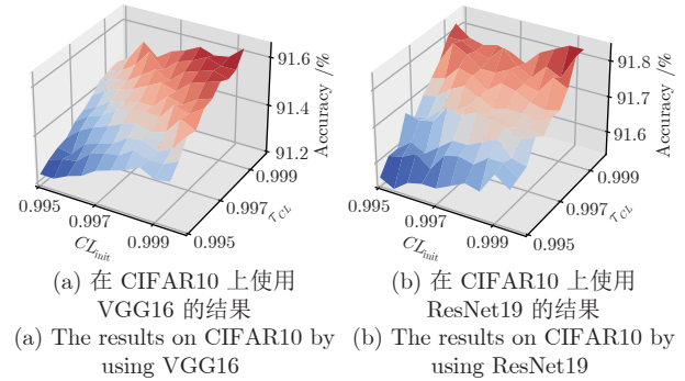
图 5 超参数对准确率的影响
