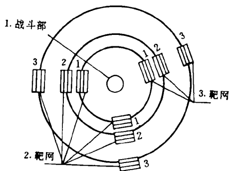
图 1 靶网测速试验场地布置图
