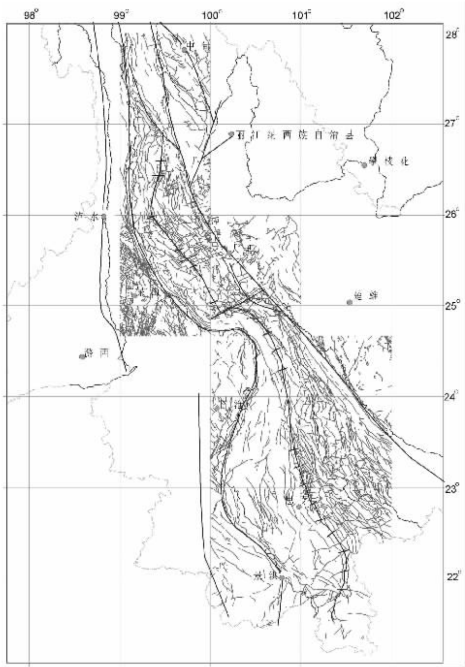
图 1 兰坪—思茅盆地断裂构造分布(据 1:20 万数字地质图修编)
