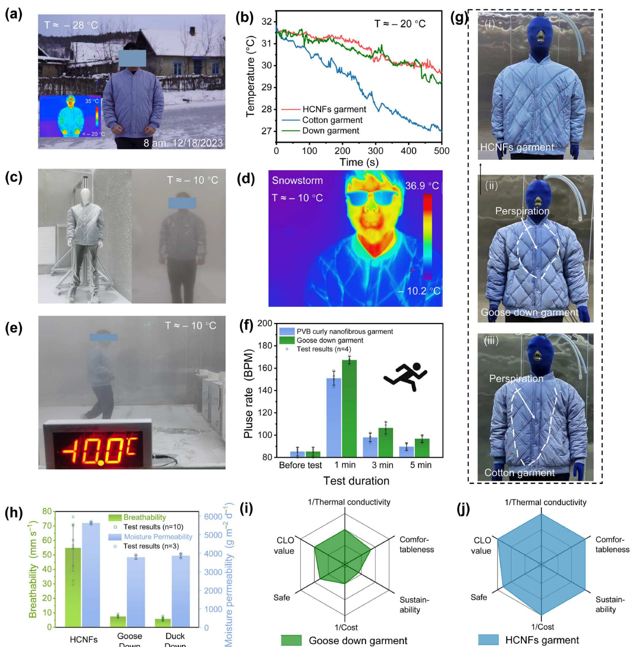
图 2 (网络版彩色)超保暖纳米纤维服装. (a) -28^{\circ}\text{C} 高纬度地区(北纬 53.5^{\circ} )穿着HCNF服装的光学图像及红外热像图; (b) -20^{\circ}\text{C} 环境下不同厚度服装(HCNF、棉质、850蓬松度鹅绒)的温度传感实验; (c) 出汗假人法与暴风雪条件真人试验评估HCNF服装保暖性; (d) -10^{\circ}\text{C} 暴风雪条件下穿着HCNF服装的红外热像图; (e) -10^{\circ}\text{C} 暴风雪条件下穿着HCNF服装的运动记录; (f) 穿着鹅绒与HCNF服装的运动后心率变化分析( n=4 , 平均值 \pm 标准差); (g) 不同保暖服装汗液浸泡实验的防水性评估; (h) HCNF服装内衬与鹅绒、鸭绒的透湿性( n=3 , 平均值 \pm 标准差)及透气性( n=10 , 平均值 \pm 标准差)对比; (i), (j) 鹅绒服装与HCNF服装的六维性能对比分析 [3] . Reproduced with permission from Springer Nature
