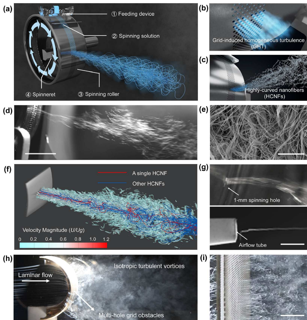
图 1 (网络版彩色)GHTS装置生成的湍流诱导弯曲纳米纤维。(a) GHTS 装置示意图; (b) 网格诱导均匀湍流(GHT)形成的示意图; (c) GHTS装置大规模生产HCNFs的示意图; (d) GHTS 系统制备HCNFs的高速摄像图像(比例尺: 20 mm); (e) GHTS系统生产的HCNFs的扫描电子显微镜(SEM)图像。比例尺: 20 \mu\text{m} 。 (f) GHT作用下气流速度与纳米纤维卷曲的计算流体力学(CFD)模拟结果( U 为实际速度, U_g 为气流喷嘴出口平均速度); (g) 相同能耗下GHTS与溶液吹纺(SBS)系统纺丝溶液射流对比(比例尺: 5 mm); (h), (i) 流场可视化图像(比例尺: 1 cm) [3] 。 Reproduced with permission from Springer Nature
