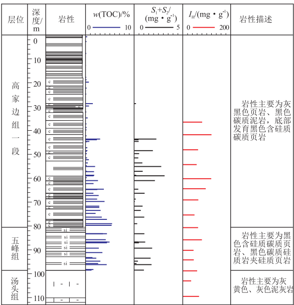
图6 安徽巢湖地区DC1井上奥陶统五峰组—下志留统高家边组烃源岩综合柱状图
