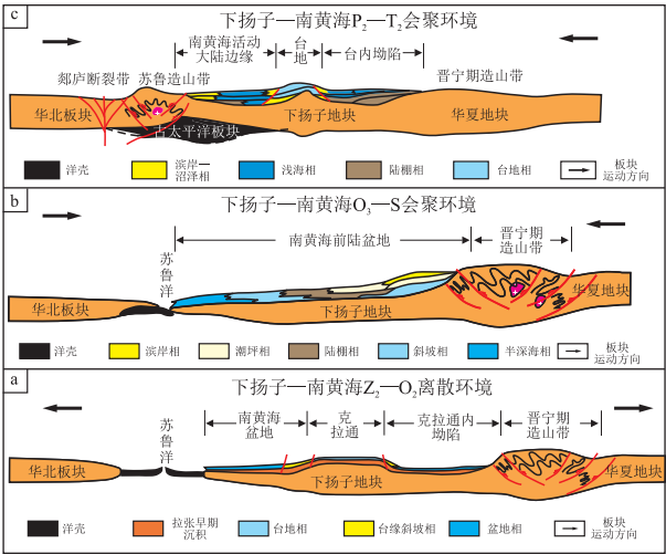
图2 南黄海地区古生代盆地原型类型 据文献[1,30-32]修改。 Fig.2 Paleozoic basin type in South Yellow Sea area
