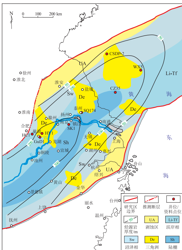
图7 下扬子—南黄海地区上二叠统龙潭组岩相及烃源岩分布
