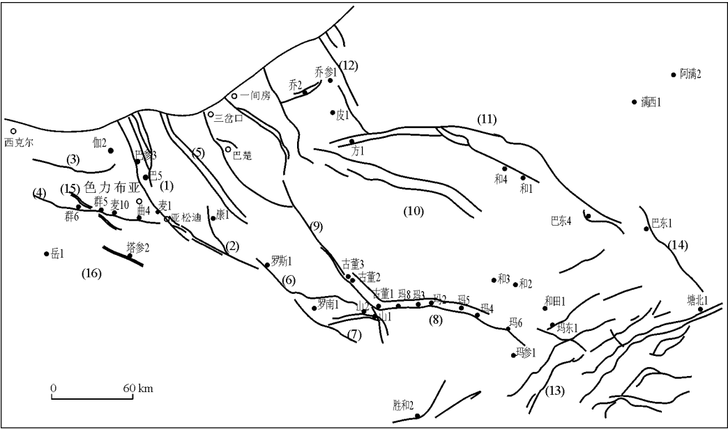
图 2 塔里木西部巴楚—麦盖提地区的主要断裂 [21] (1)色力布亚;(2)康塔库木;(3)阔什拉克;(4)巴什托普;(5)曲许盖;(6)罗斯塔格;(7)鸟山;(8)玛扎塔格; (9)古董山;(10)卡拉沙依;(11)吐木休克;(12)阿恰;(13)玛东;(14)巴东;(15)巴西;(16)塔参 2 井南
