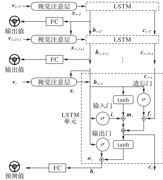
图3 LSTM层结构
