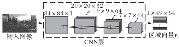
图2 CNN层结构
