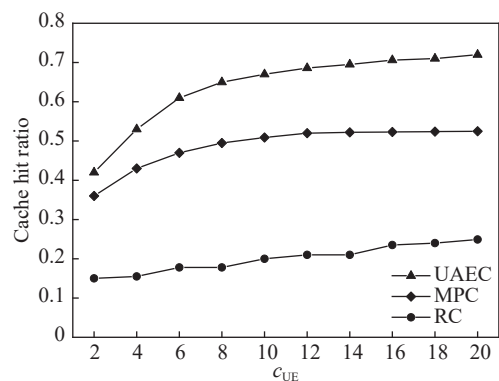
图 4 不同机制中缓存命中率随着缓存容量的变化 Fig.4 Cache hit ratio versus cache capacity in different mechanisms
