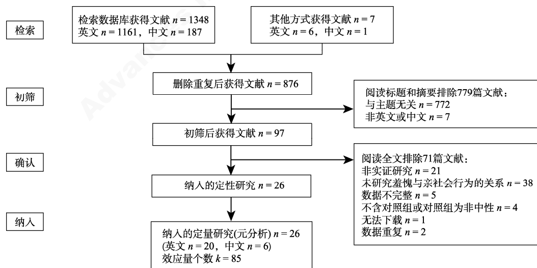
图1 PRISMA流程图
