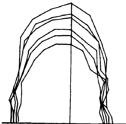
图 6 用 TP-5 型得的数据由绘图仪绘制的 Fig. 6 Profile drawn by plotting instrument using TP-5 type interpretroscope
