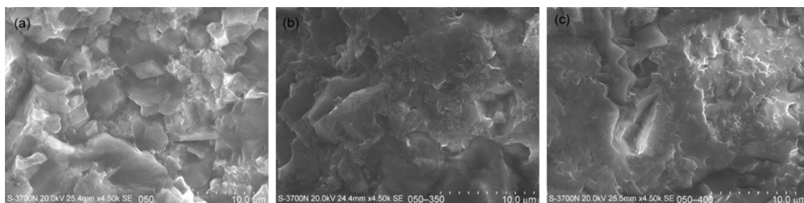
图 6 050 实验标本热处理前后扫描电子显微镜对比
