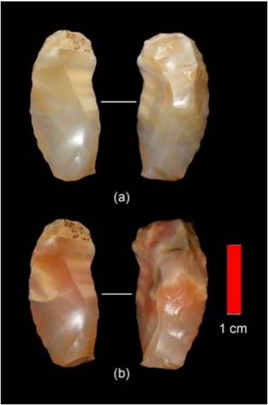
图 4 室内实验燧石标本热处理前后对比 (a) 热处理前; (b) 热处理后
