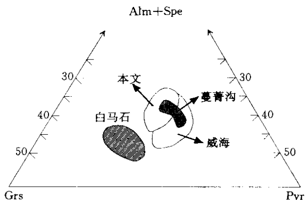
图2 高压麻粒岩石榴石的 (Alm+Spe)-Pyr-Grs 图解 Fig. 2 (Alm+Spe)-Pyr-Grs diagram for garnets from high-pressure mafic granulites
