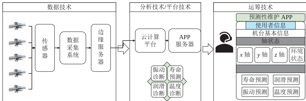
图 3 滚珠丝杠维护系统工业应用架构图
