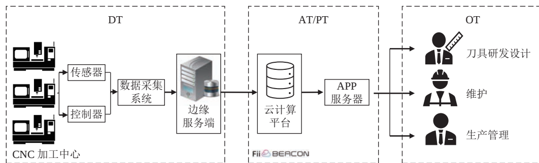
图8 刀具寿命监控及预测技术构架图
