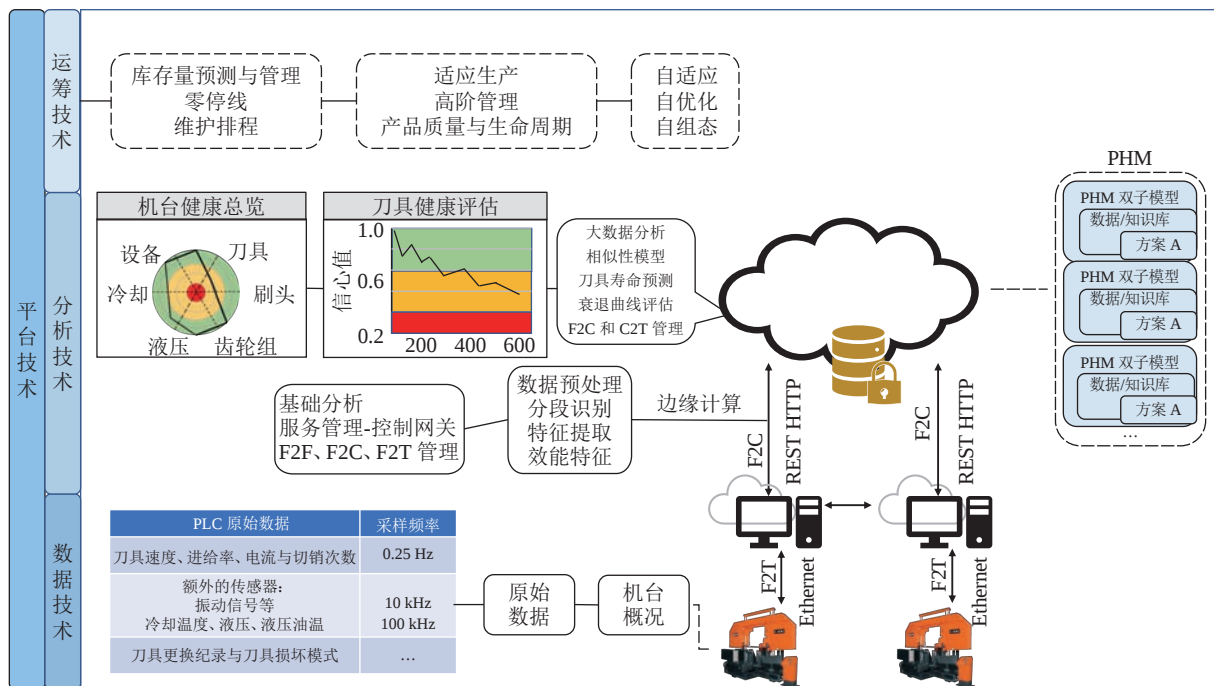
图 5 工业人工智能在刀具智能制造系统上的应用
