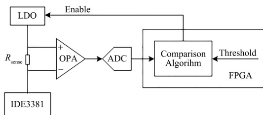
图6 电流监控模块框图
