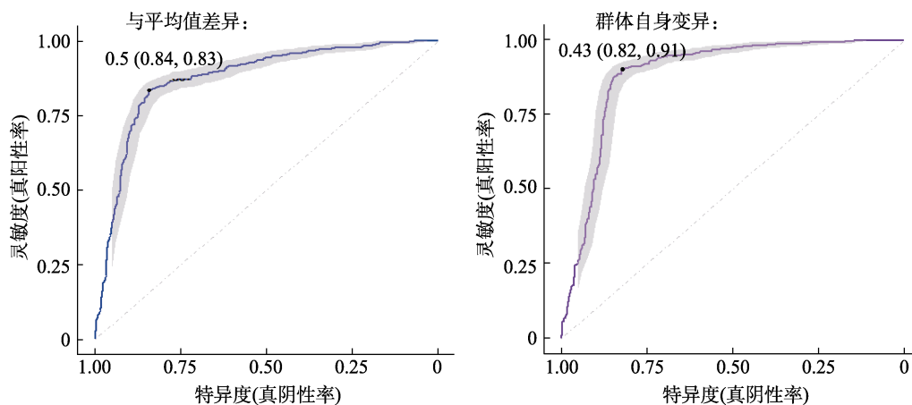
图 3 实验 1 中模型拟合的接收者操作特征曲线 (ROC 曲线)
