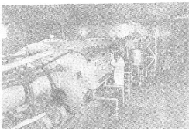
图 3 建成后的 SSC
