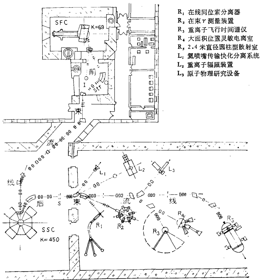
图 1 兰州重离子加速器系统图
