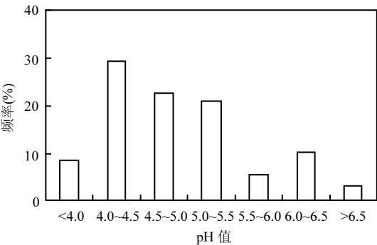
图2 三峡库首地区降水 pH 值频率分布特征 Fig.2 Frequency distribution of pH
