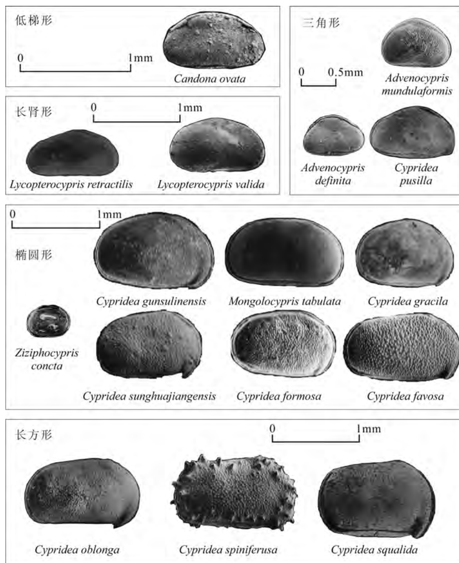
图6 松辽盆地姚家组—嫩江组一段介形类壳形类型
