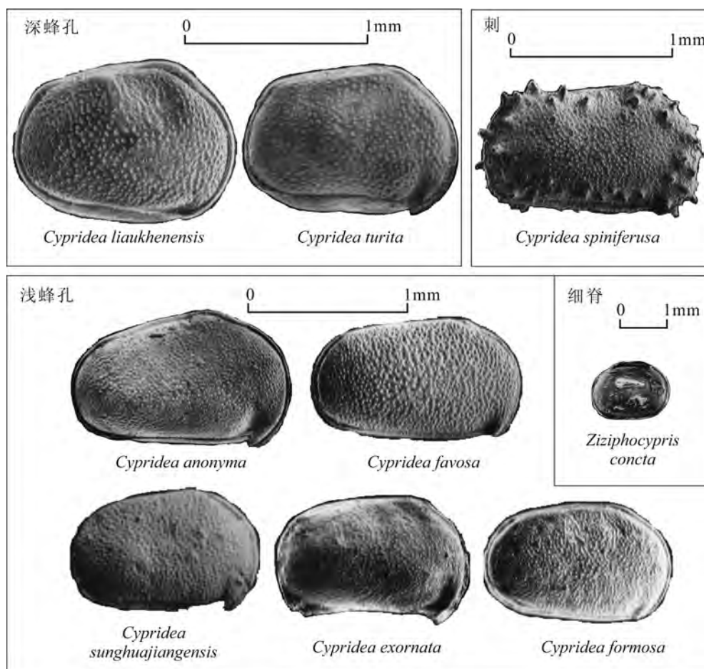
图3 松辽盆地姚家组—嫩江组一段介形类壳饰类型
