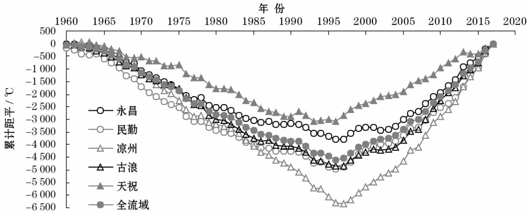
图 5 石羊河流域≥10℃积温的累计距平
