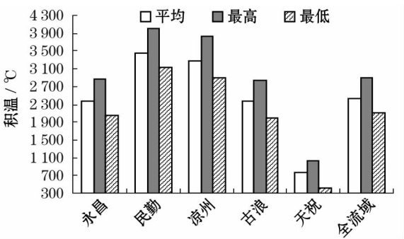
图 2 石羊河流域 \geq 10\text{ }^{\circ}\text{C} 积温平均和极值
