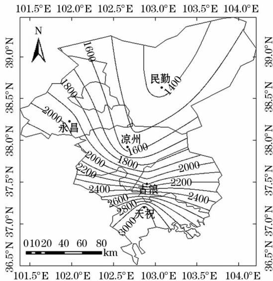
图1 石羊河流域气象站点和海拔高度空间分布
