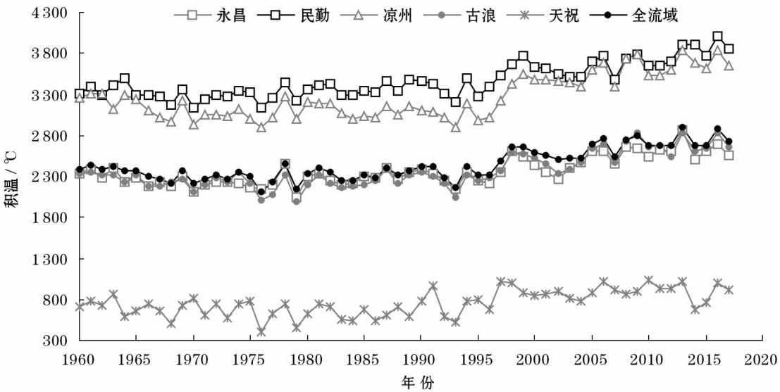
图 3 石羊河流域 \geq 10\text{ }^{\circ}\text{C} 积温年变化
