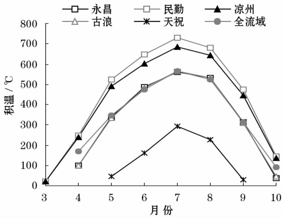
图 4 石羊河流域≥10℃积温月变化
