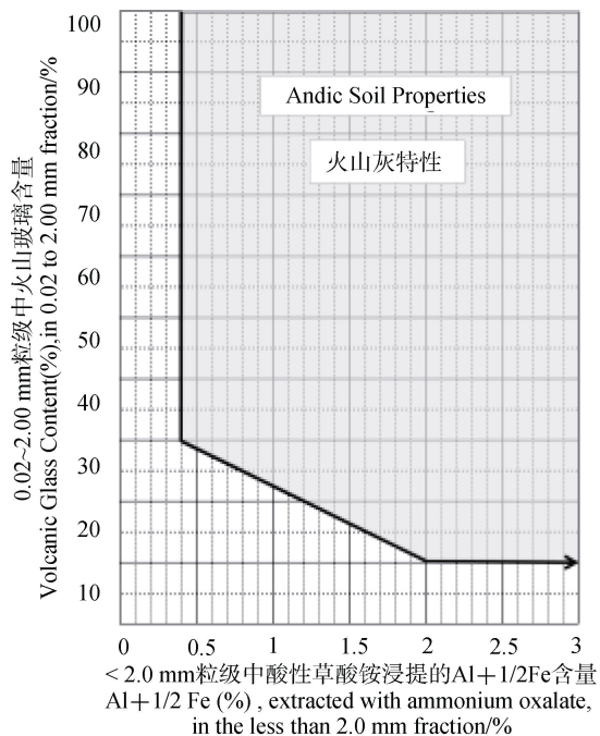
图 1 火山灰特性与 \text{Al} + 1/2\text{Fe} 含量和火山玻璃含量的关系图
