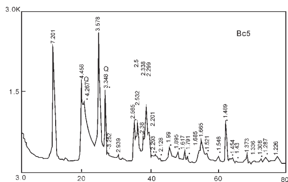
图2 广西南宁地区球粘土的X射线衍射分析曲线 (主要为无序高岭石,次为少量石英)
