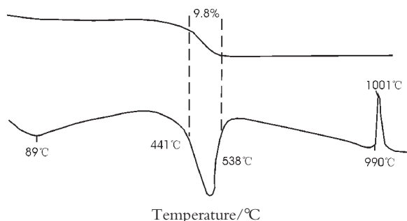
图1 广西南宁地区球粘土的综合热分析曲线
