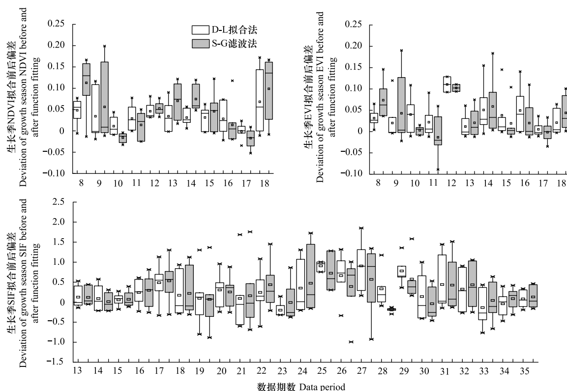
图5 3种指数拟合前后残差箱线图(只保留生长季(4—9月)高质量数据点)
