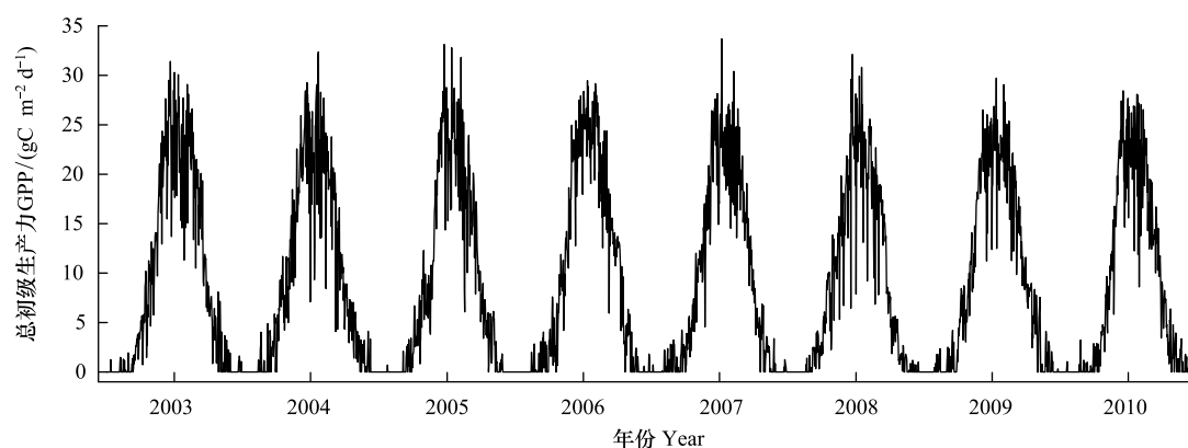
图2 长白山站 2003—2010 年 GPP 季节变动曲线图
