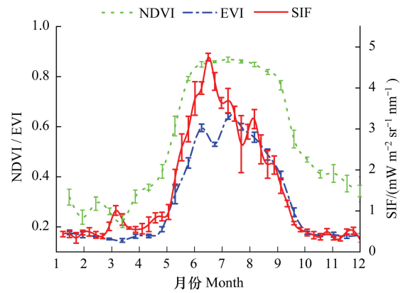
图 7 3 种指数 7 年均值时间序列曲线
