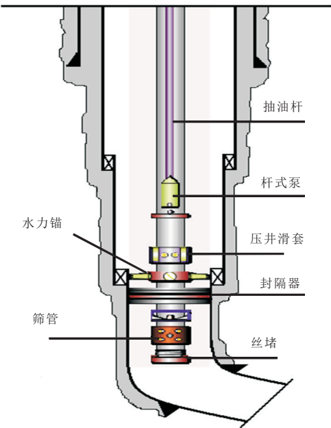
图 1 卡封管柱治理套损工艺示意 Fig.1 Sealing of casing damage
