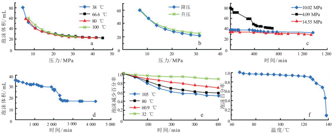
图2 泡沫剂和稳定性关系 据参考文献[4]。
