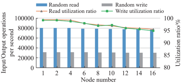
图10 共享存储系统 IOPS 性能分析
