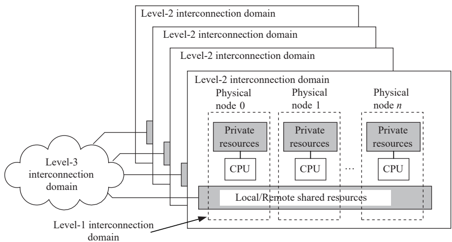
图4 分布式云服务器结构
