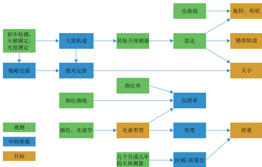
图1 近地物体表征过程 [5]
