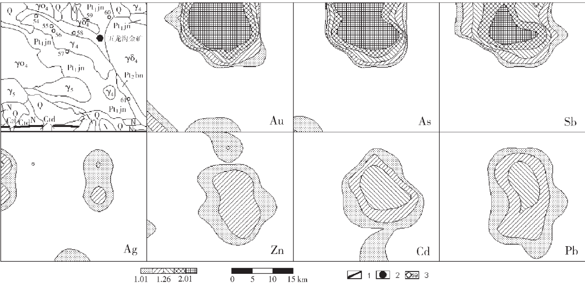
图 1 青海省五龙沟金矿衬值异常图
