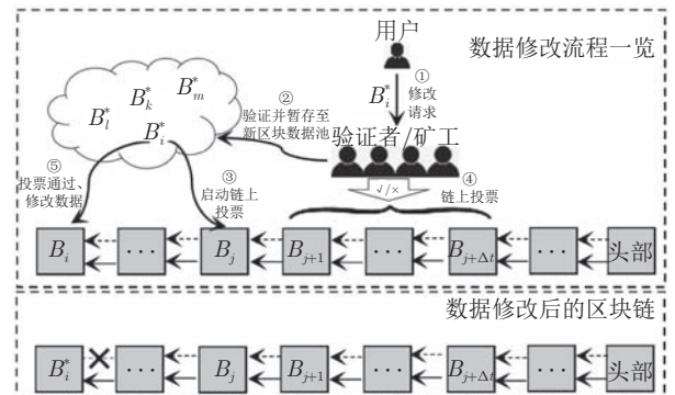
图 4 基于平行双哈希链的数据修改流程
