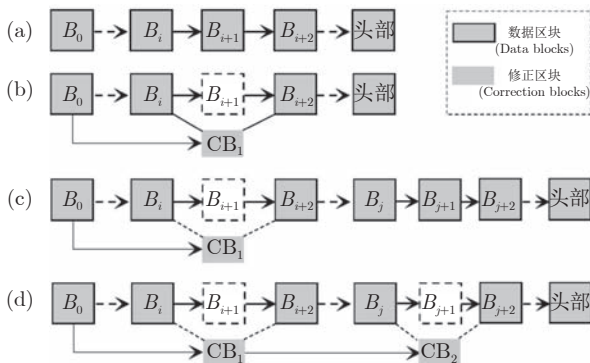
图 3 基于平行双区块链的数据修改流程
