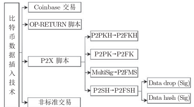
图 6 比特币数据插入技术框架
