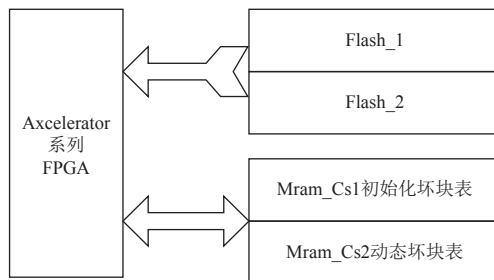
图2 坏块表存储示意图
