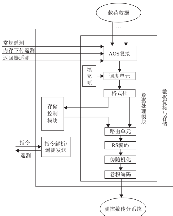
图1 大容量固定及复接模块的信息流程框图
