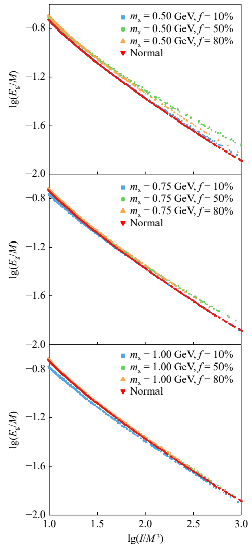
图 6 E_g/M-I/M^3 关系曲线 (坐标均取对数)
