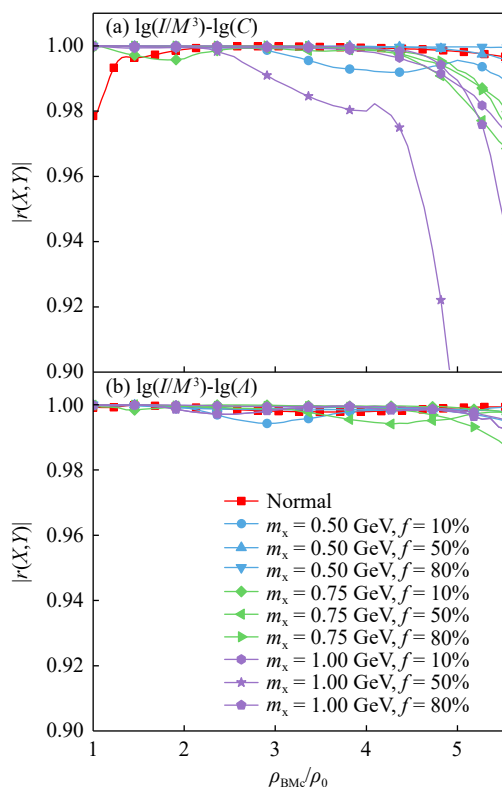
图 4 无量纲转动惯量 I/M^3 与不同性质参量间的关联度 (在线彩图)
