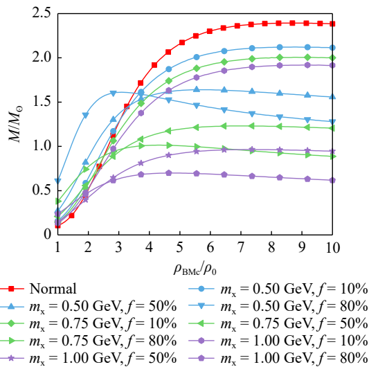
图 2 核物质物态为 APR3 时的 M-\rho_{\text{BMc}} 关系图 (在线彩图)
