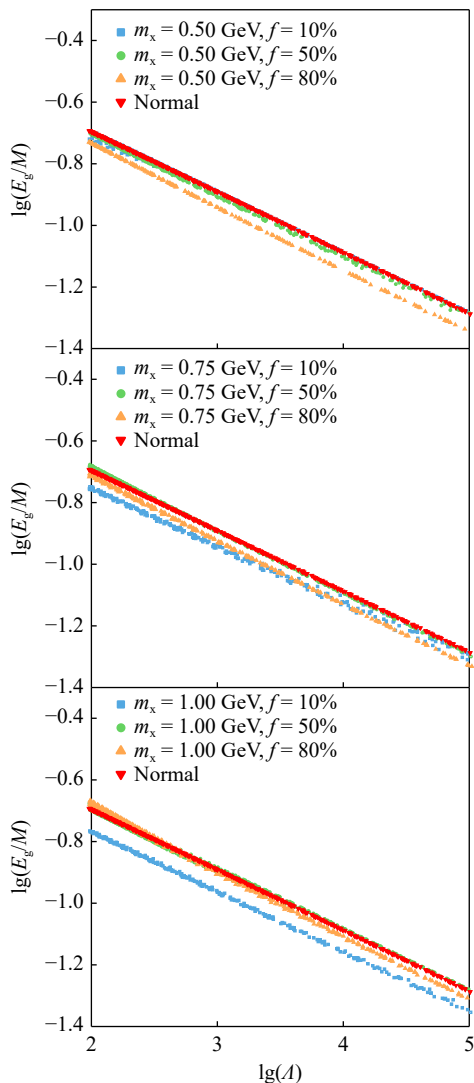
图 5 E_g/M-A 关系曲线 (坐标均取对数)
