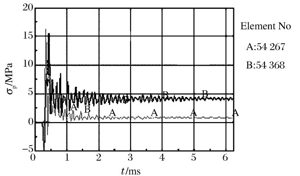
图 3 炮孔横向中心线上两单元应力时程曲线
