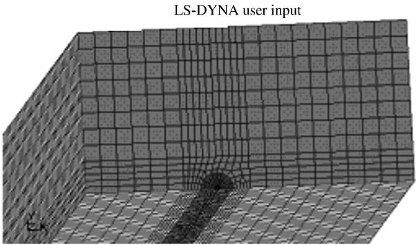
图 1 模型剖面网格划分图
