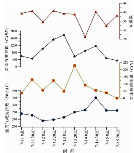
图6 郴州站2006年7月11–15日大气不稳定指数
