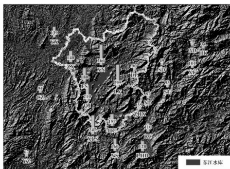
CZ = 郴州; FS = 方石; GD = 桂东; HC = 黄草; HK = 寒口; LHD = 龙虎洞; LP = 连坪; LX = 龙溪; ND = 南洞; QJ = 清江; RC = 汝城; SD = 四都; ST = 沙田; XF = 新坊; XLS = 秀里山; XN = 兴宁; YS = 延寿; YX = 永兴; YZ = 宜章; ZHX = 樟溪; ZX = 资兴 图3 研究区 2006 年 7 月 14 日 20:00–15 日 08:00 各站 12 h 累计雨量
