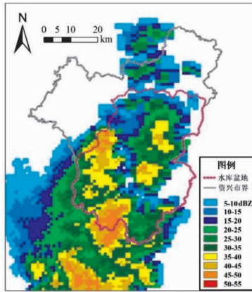
图4 2016年7月14日23:00研究区雷达回波(1.5°仰角)
