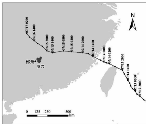
图2 碧利斯最佳路径
