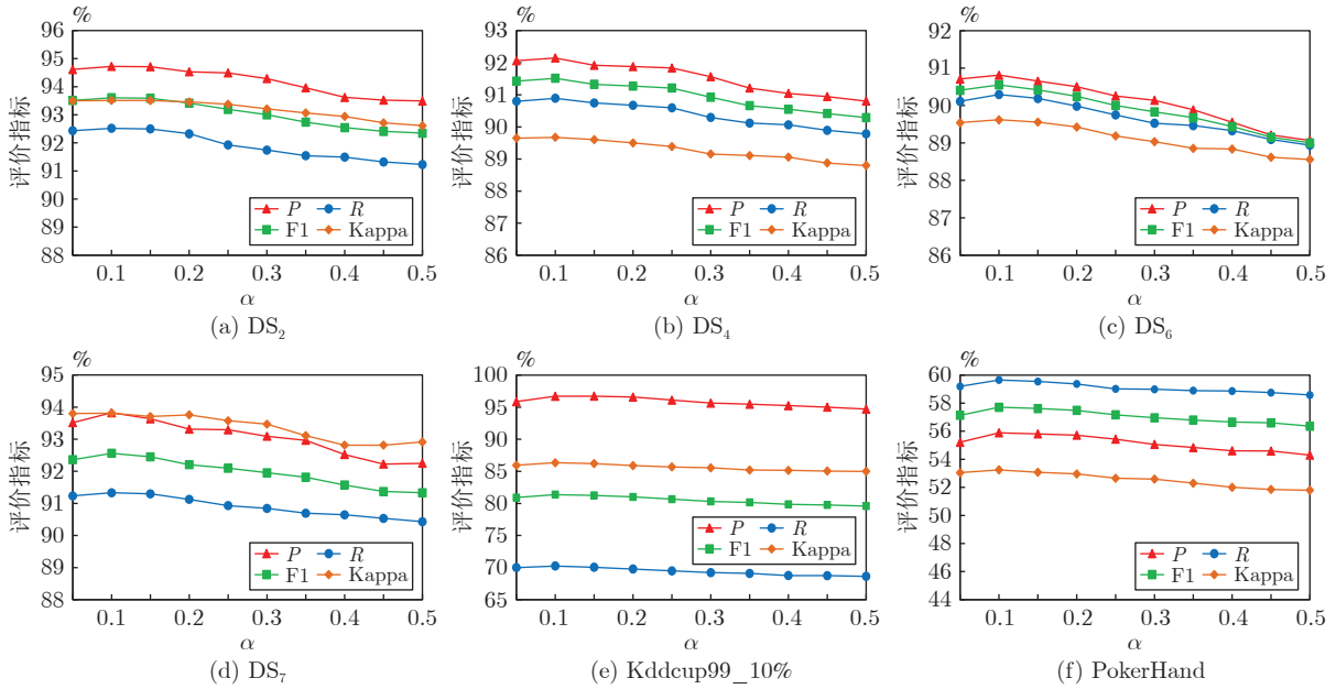
图 8 参数 \alpha 对算法的影响
