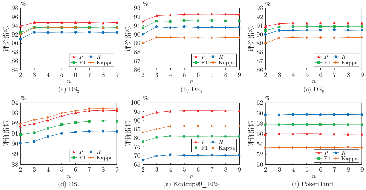
图 7 参数 n 对算法的影响
