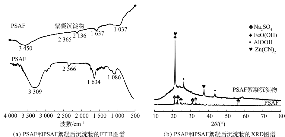
图 6 PSAF 和 PSAF 絮凝后沉淀物的 FTIR 图谱和 XRD 图谱
