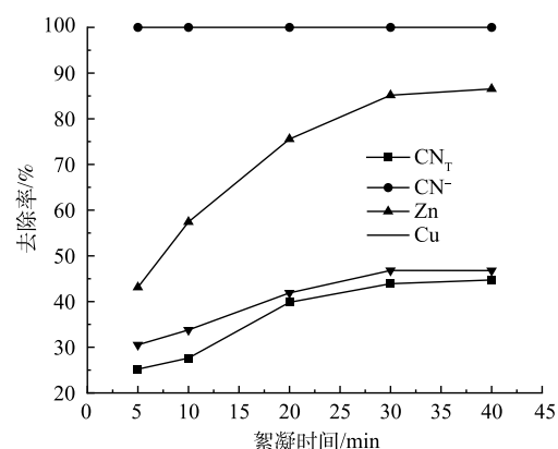
图 5 絮凝时间对去除率的影响
