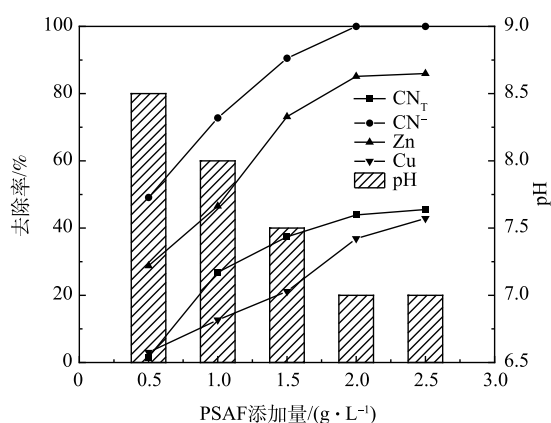
图2 PSAF添加量对去除率的影响及pH的变化
