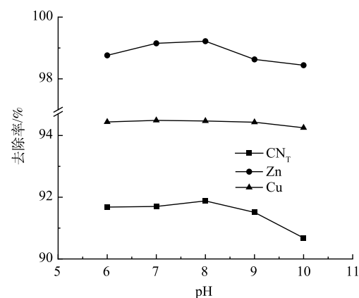
图 10 pH 对去除率的影响
