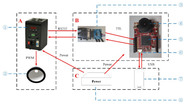
注: A. 灯组和其控制器电路; B. 串口通信模块和 CMOS 相机及其控制电路; C. 系统的独立电源以及智能手机外设; ①为灯组控制器; ②为激发光灯组; ③为串口通信模块; ④为 CMOS 相机; ⑤为微控制单位 MCU; ⑥为 USB 接口; ⑦为智能手机外设; ⑧为独立电源
