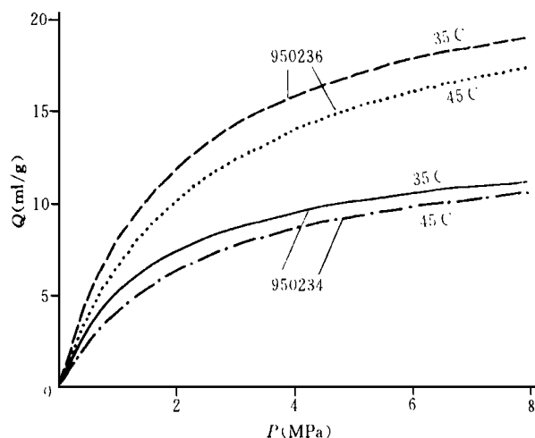
图 1 不同温度下等温吸附曲线
