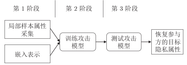
图4 VFL中协作方的攻击流程
