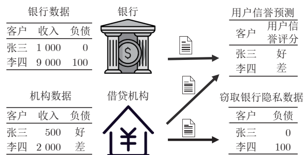
图1 VFL隐私泄露示例
