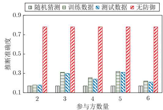
图 11 PPVFL 在多个参与方场景下隐私保护的性能
