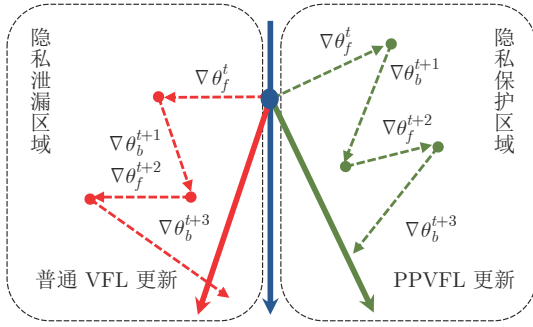
图 6 防御方法示意图
