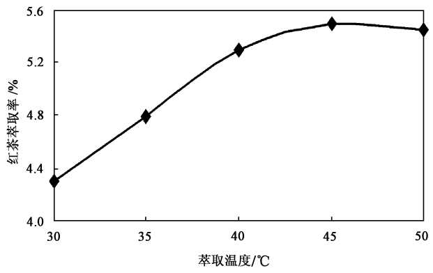
图 4 萃取温度对红茶萃取率的影响
