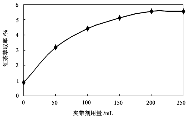
图 3 夹带剂用量与红茶萃取率的关系
