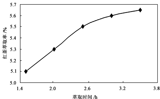
图1 萃取时间对红茶萃取率的影响
