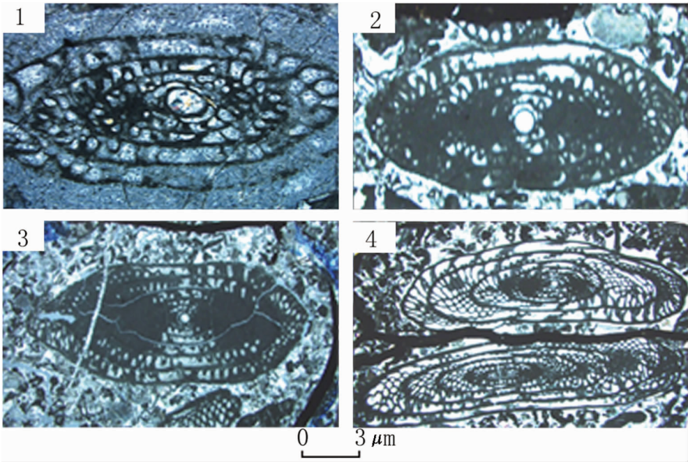
图 5 早—中二叠世地层鲃化石 Fig.5 Early-Mid Permian fusulinids
