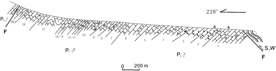
图 3 新疆和田市岔路口地区红山湖一带早—中二叠世地层实测剖面图 F—断层; P_{1-2}^1 —下—中二叠统下段; P_{1-2}^2 —上—中二叠统上段
