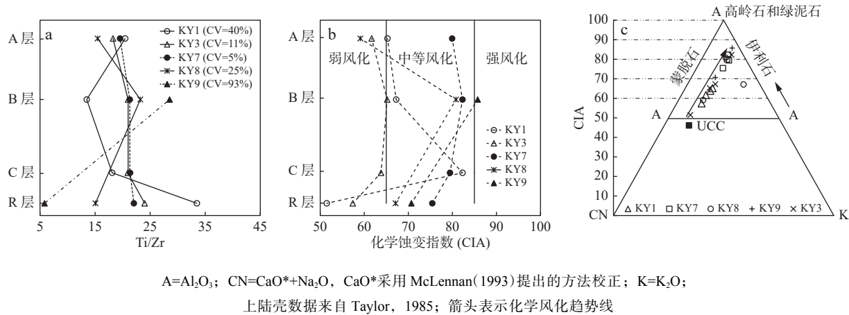
图3 不同岩石风化剖面 Ti/Zr 值剖面分布、变异系数(a)及各发生层化学蚀变指数(b)和 A-CN-K 三角图解(c) Fig. 3 (a) The distribution and (b) coefficients of variation of Ti/Zr ratios and (c) A-CN-K ternary diagrams in different rock weathering profiles
