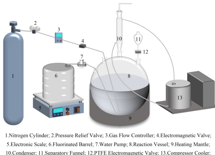
图1 湿法氧化装置示意图 Fig.1 Schematic of the wet-oxidation system
