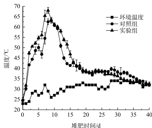
图2 堆肥过程中堆体温度变化
