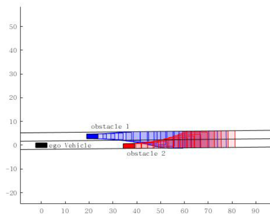
图 15 场景图 13(c)的占有率
