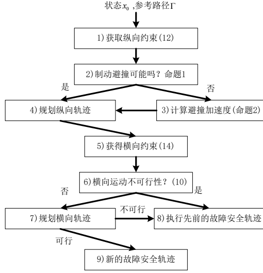
图6 故障安全轨迹计算步骤 [58]
