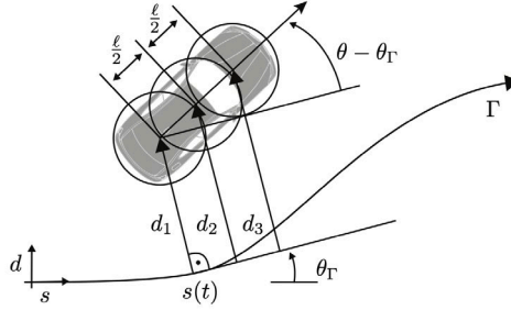
图 5 曲线坐标系下的运动模型 [58]
