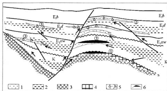
图 4 汤原断陷油气成藏模式
